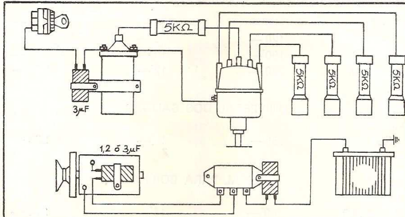
EJEMPLO DE PROTECCION ANTIPARASITARIA EN AUTOMOVILES EQUIPADOS CON DINAMO.
